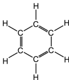
Benzene Ring
